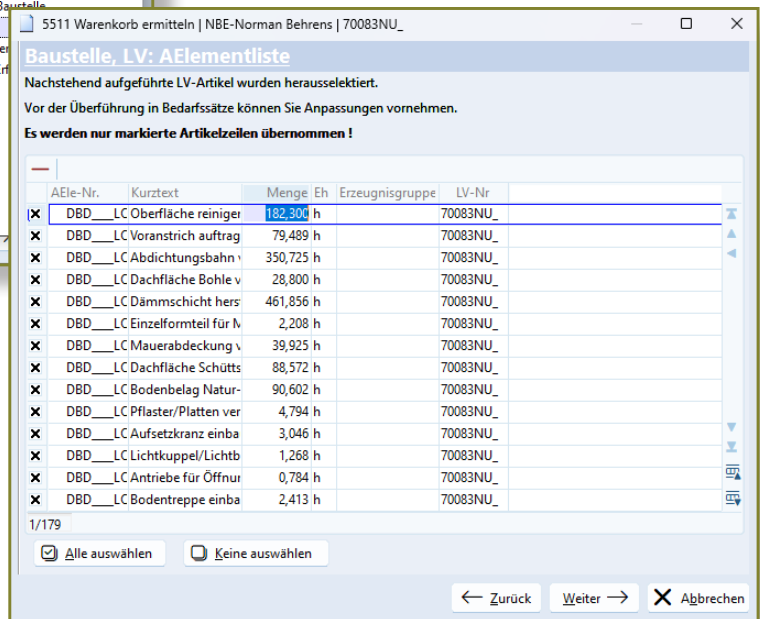
Abb. 3: Ermittelter Bedarf
