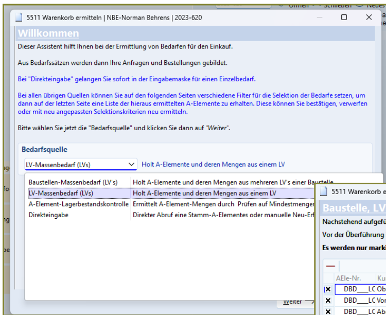
Abb. 2: Startbildschirm Bedarfsermittlung
